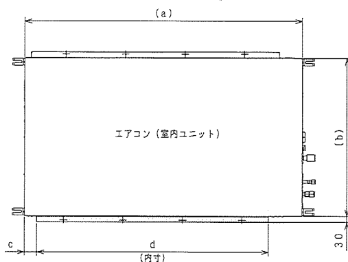
取付状態図
